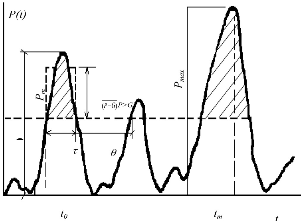
Рис. 1. Пересечение траекторией случайного процесса P(t) критического уровня G Fig. 1. The intersection of the trajectory of a random process P(t) critical level G
