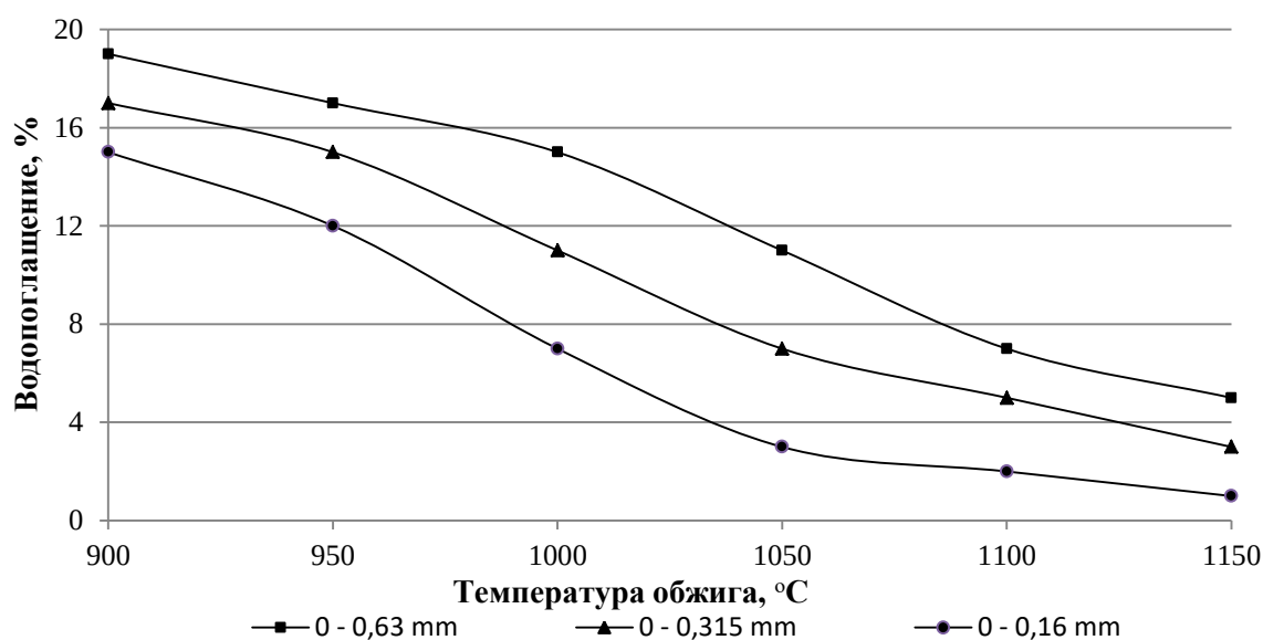
Рис. 4 Влияние степени измельчения и температуры обжига на водопоглощение образцов Fig. 4 The influence of the degree of grinding and the firing temperature on the water absorption of samples
