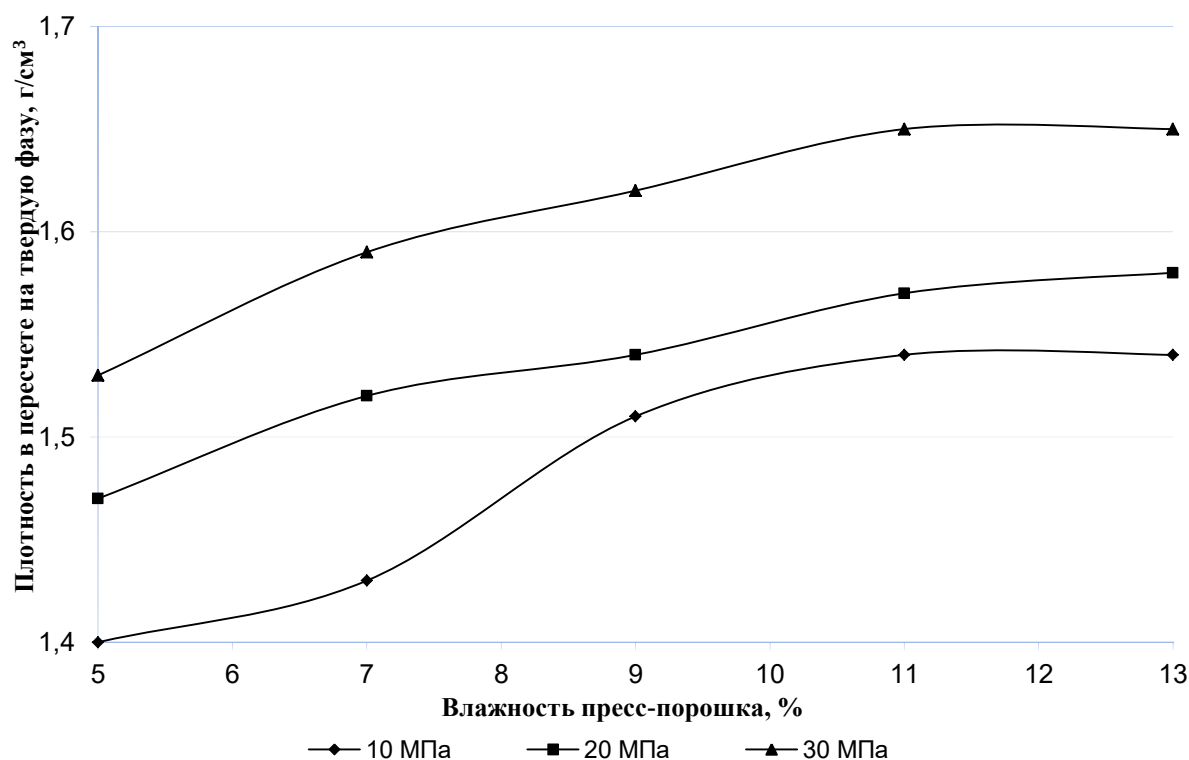
Рис.5 Влияние влажности пресс-порошков на прессуемость образцов Fig.5 Influence of moisture of press powders on the compressibility of samples
