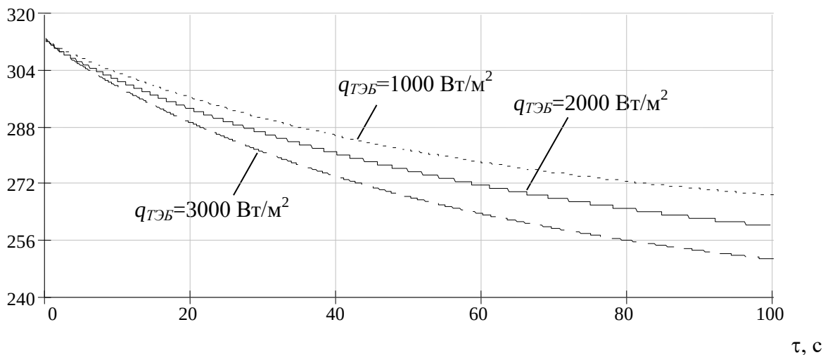
Рис. 3. Зависимость изменения температуры извлекаемого объекта от времени при различной холодопроизводительности ТЭМ
