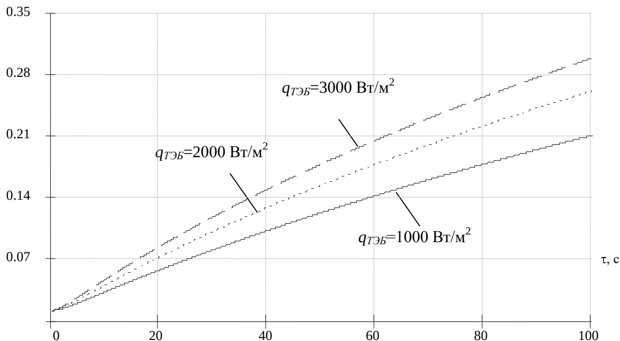
Рис. 5. Зависимость изменения толщины слоя льда от времени при различной холодопроизводительности ТЭМ
